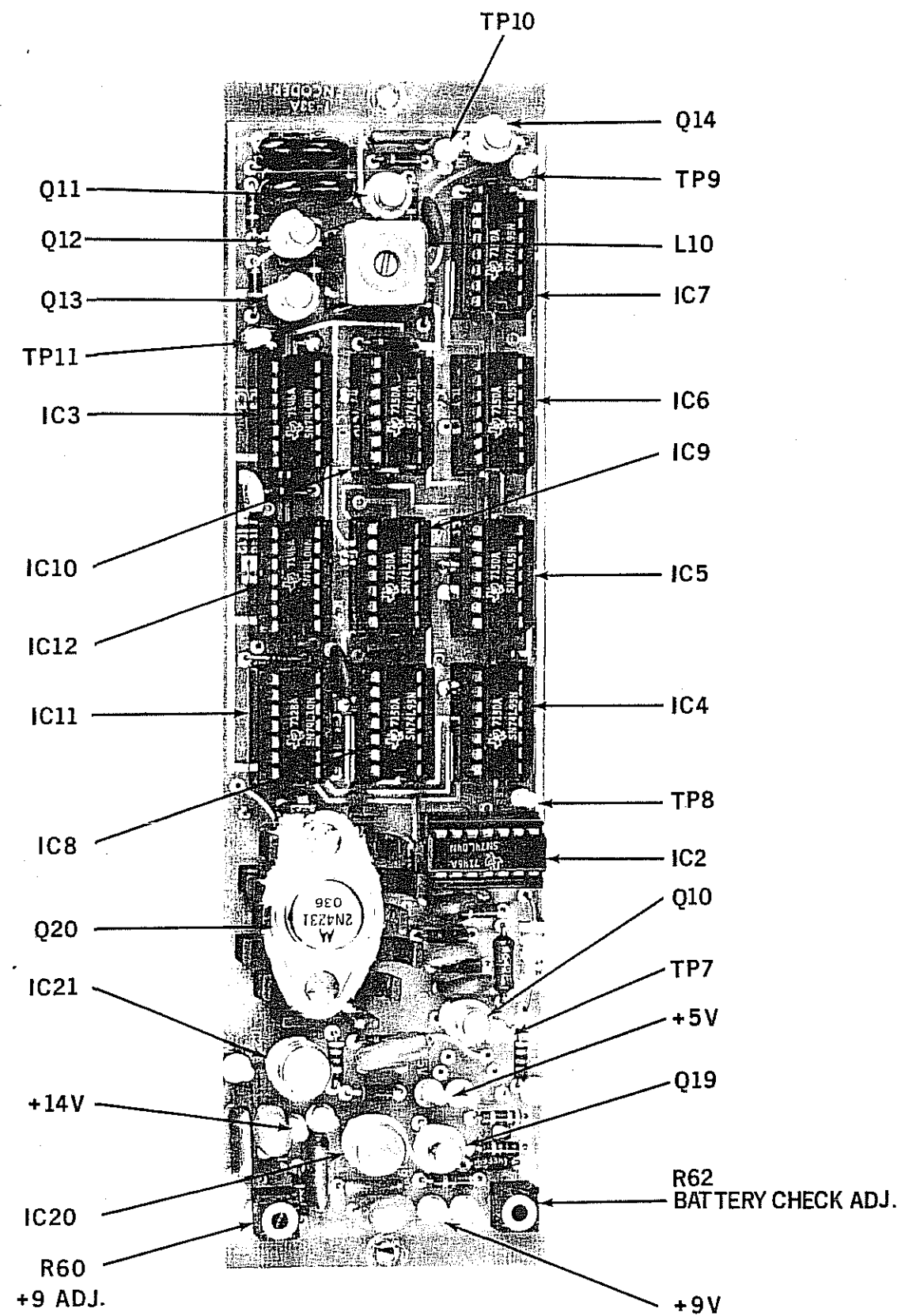
ENCODER TOP
