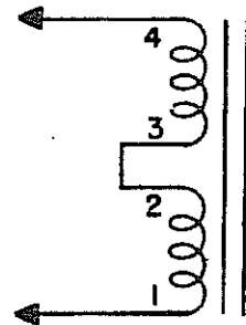
230 VOLT INPUT
