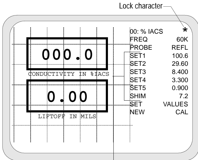
Figure 5-24. Default %IACS Display
